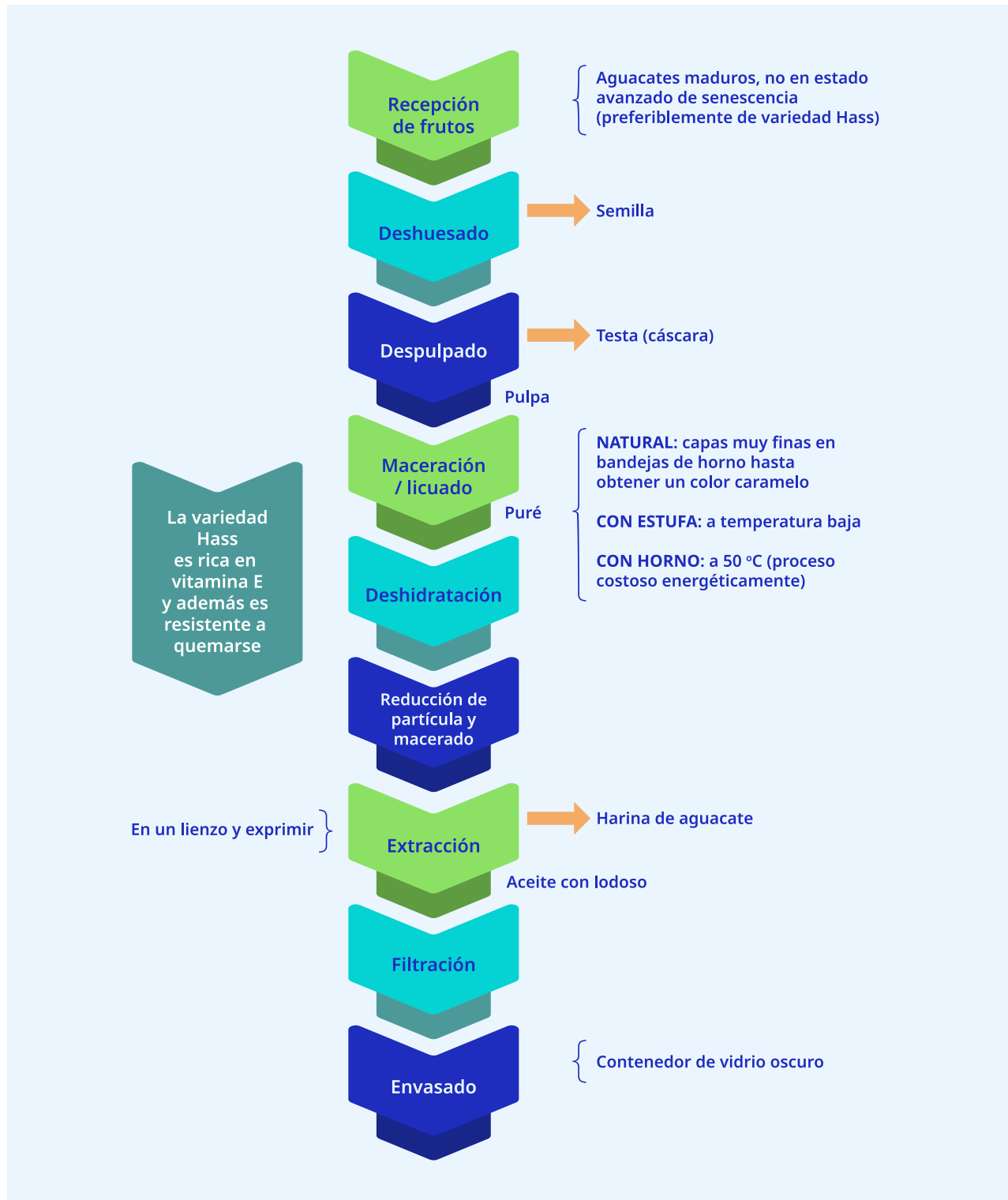
► Figura 4. Diagrama de flujo del proceso de extracción de aceite de aguacate mediante el prensado en frío
